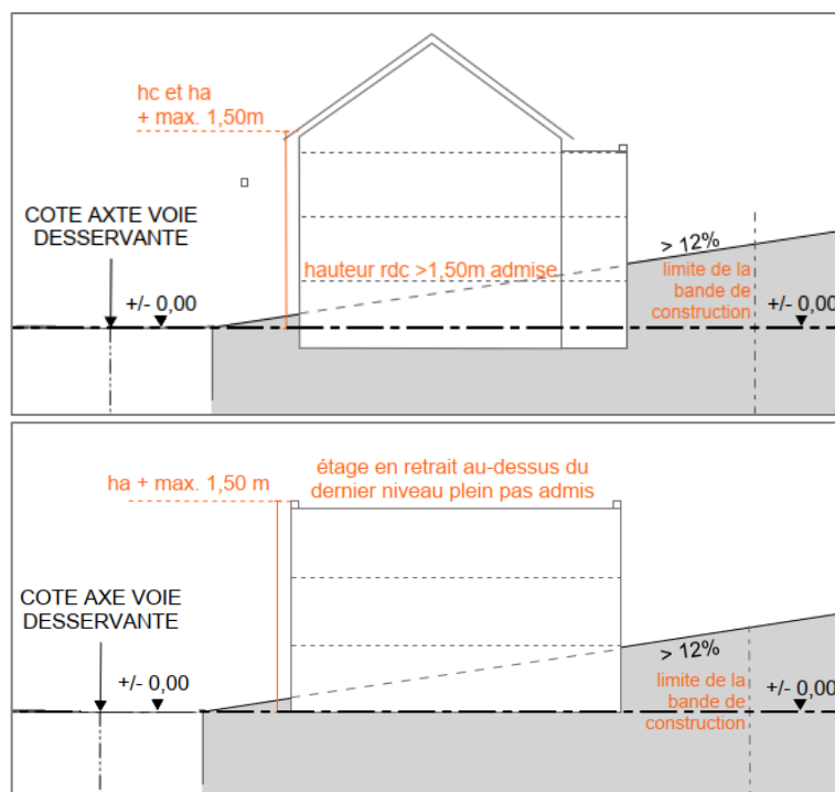
Figure 1.9.1 Terrains accidentés – dérogations terrains ascendants hc = hauteur à la corniche, ha = hauteur à l'acrotère, hf = hauteur au faîte
