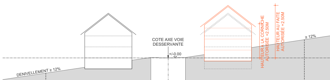
Figure 4.9.1. : Nombre de niveaux pleins admissible sur un terrain accidenté - dénivellement ascendant
