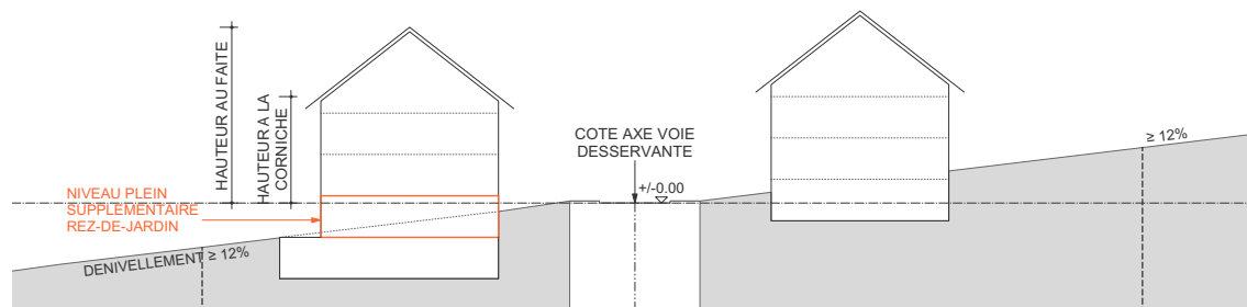
Figure 4.9.2.: Nombre de niveaux pleins admissible sur un terrain accidenté - dénivellement descendant
