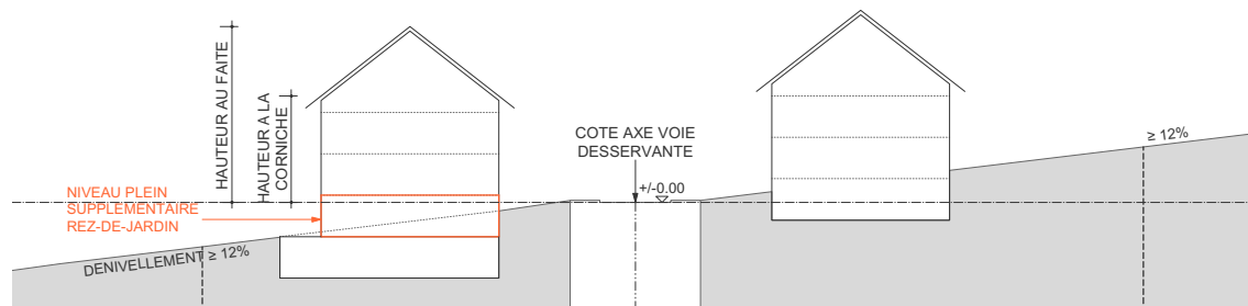
Figure 1.9.2.: Nombre de niveaux pleins admissible sur un terrain accidenté - dénivellement descendant
