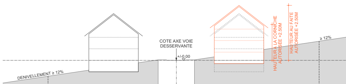
Figure 1.9.1. : Nombre de niveaux pleins admissible sur un terrain accidenté - dénivellement ascendant
