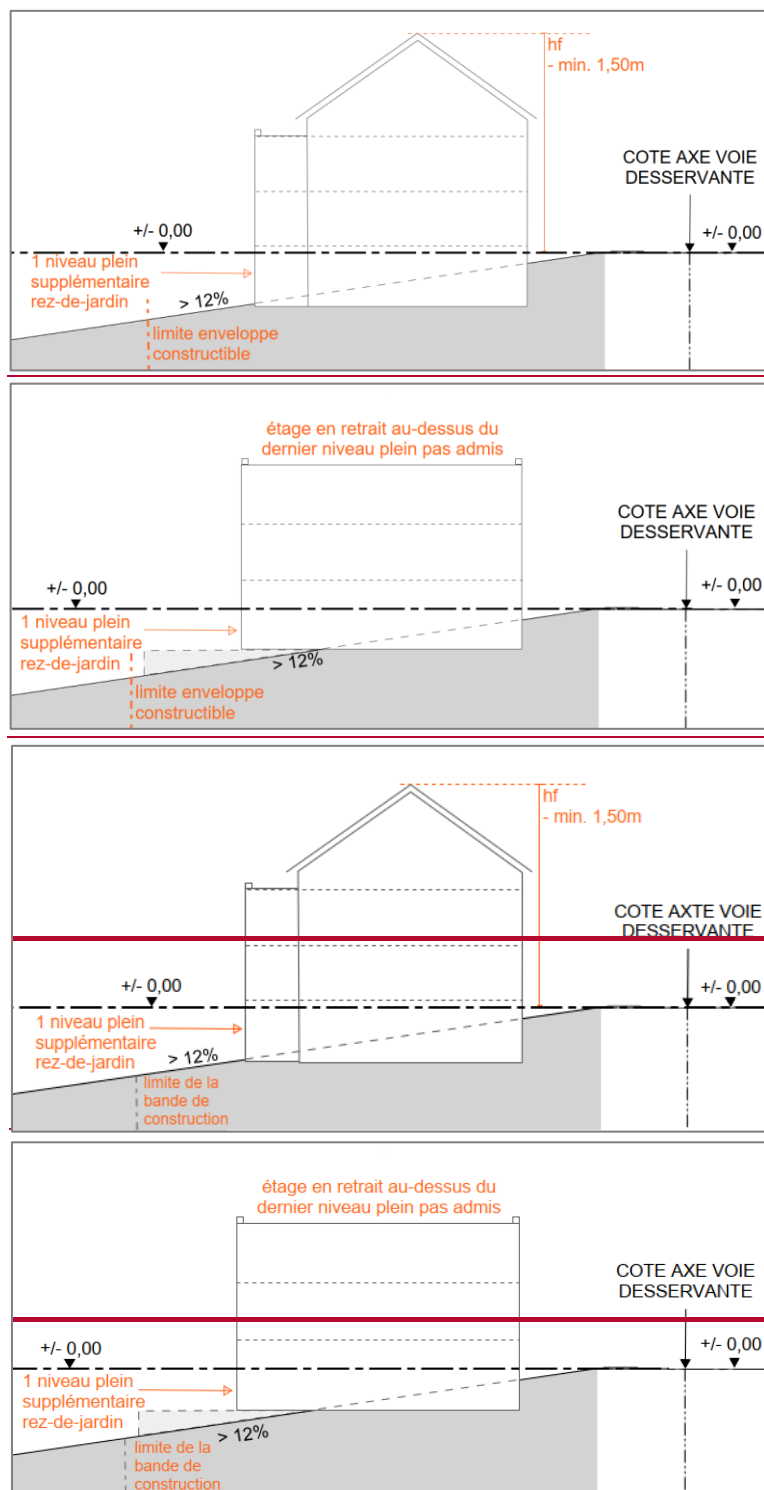
Figure 2.9.2. Terrains accidentés – dérogations terrains descendants hf = hauteur au faîte
