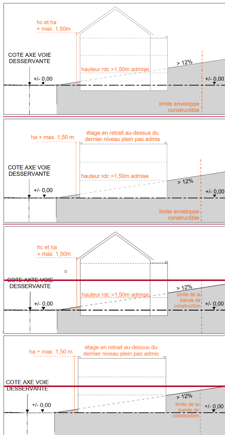
Figure 2.9.1. Terrains accidentés – dérogations terrains ascendants hc = hauteur à la corniche, ha = hauteur à l'acrotère, hf = hauteur au faîte
