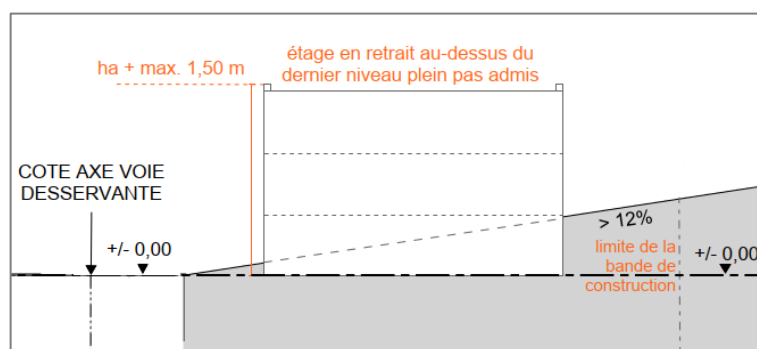
Figure 5.9.1. Terrains accidentés – dérogations terrains ascendants ha = hauteur à l'acrotère
