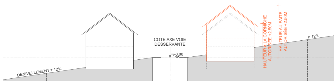
Figure 5.9.1.: Nombre de niveaux pleins admissible sur un terrain accidenté - dénivellement ascendant
