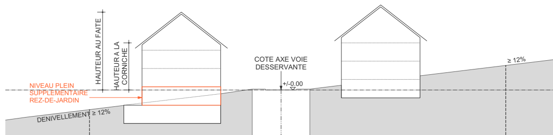
Figure 2.9.2.: Nombre de niveaux pleins admissibles sur un terrain accidenté - dénivellement descendant
