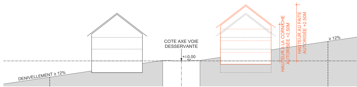
Figure 2.9.1.: Nombre de niveaux pleins admissibles sur un terrain accidenté - dénivellement ascendant
