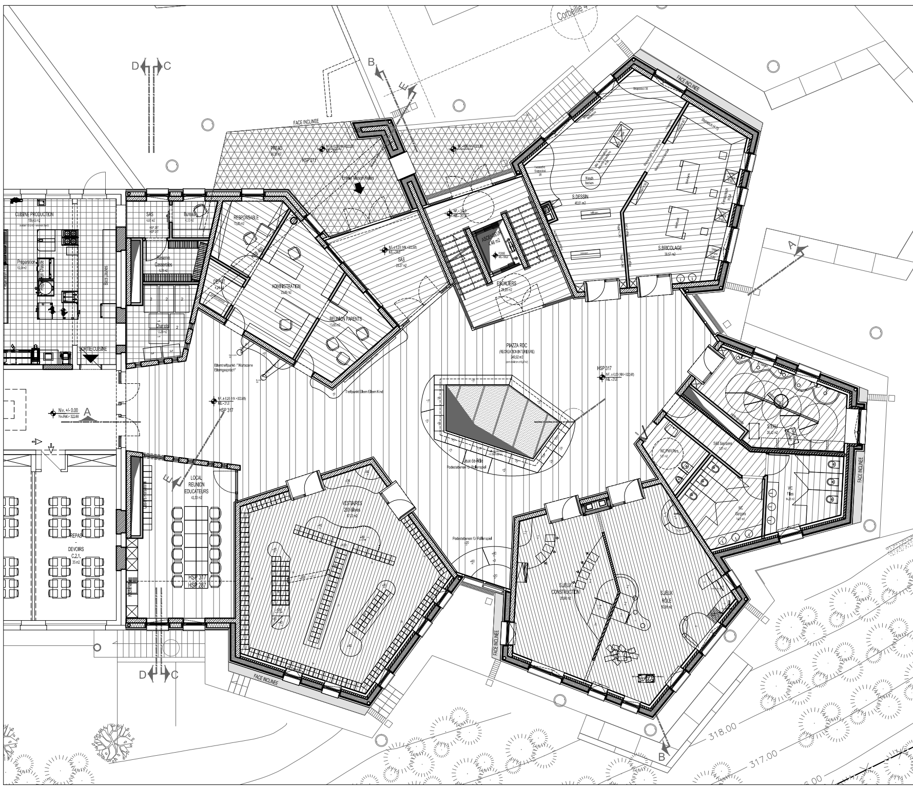
PROJET MAISON RELAIS & CYCLE C.1. 1. rue d'Ernst L-6183 Gonderange PLAN REZ-DE-CHAUSSEE
