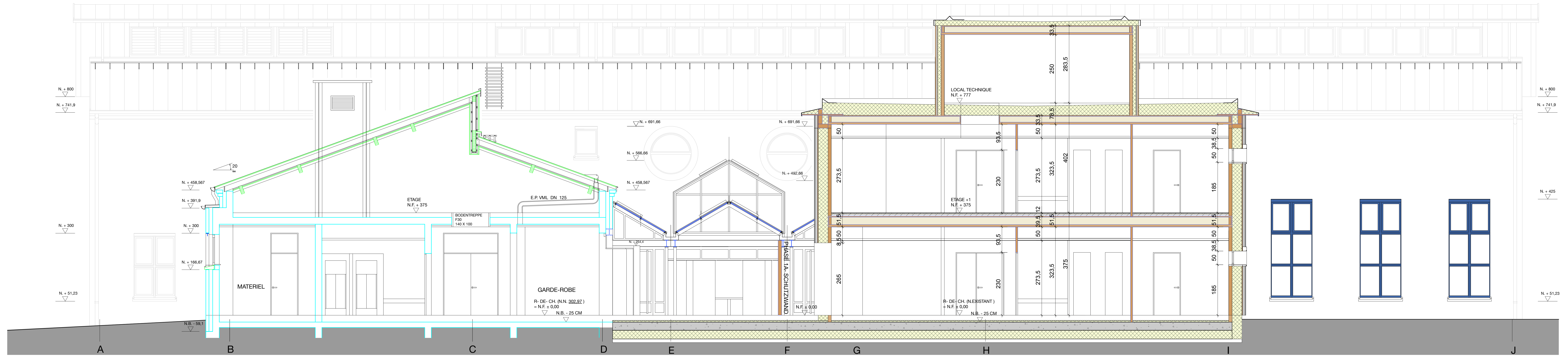
COUPE B-B - 1/50 PHASE 1A
